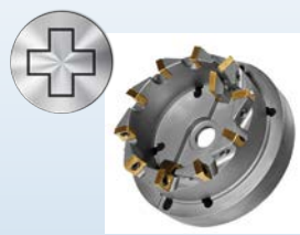
Wendeschneidplattenkronenfräser
