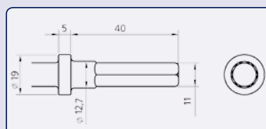
FÜR HÄMMER - RRH-2000
